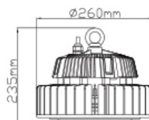
90° alu reflektor 711901 33 040 04
